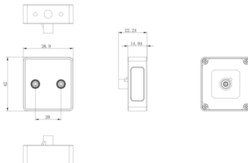
模组结构尺寸图 (38.9 × 42 × 22.24 mm)
