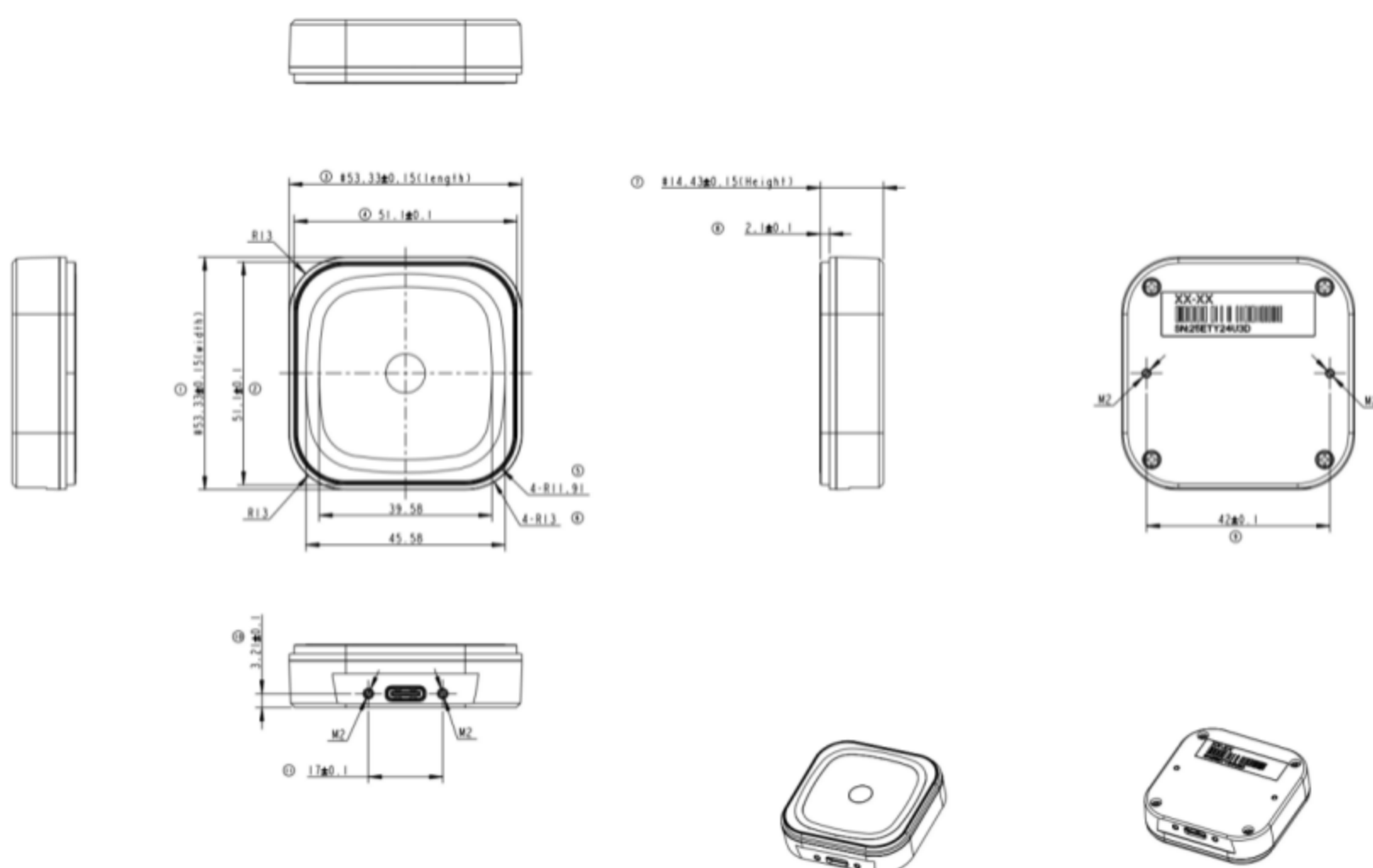
图：结构尺寸图
