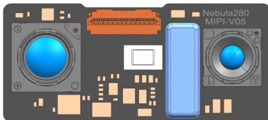
产品外观图（俯视）
