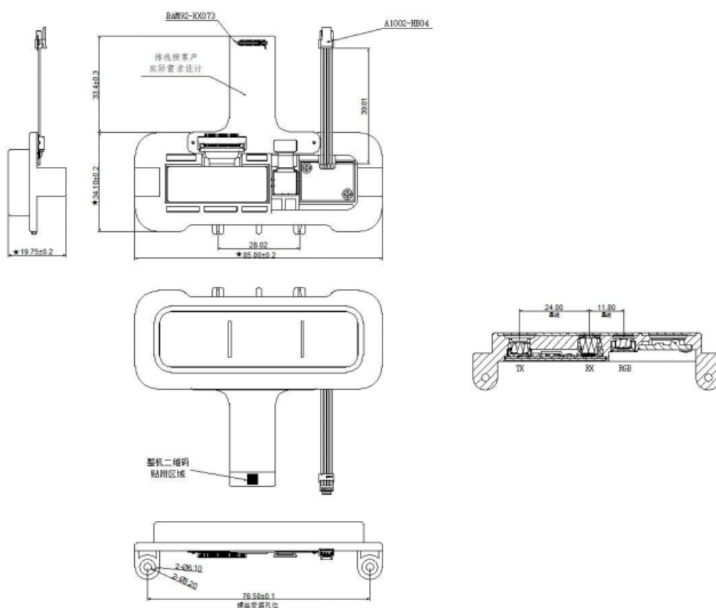
模组结构尺寸图 (含整壳装配孔位 78.50 \pm 0.1 、结构光基线 24.00、双目基线 11.80)
