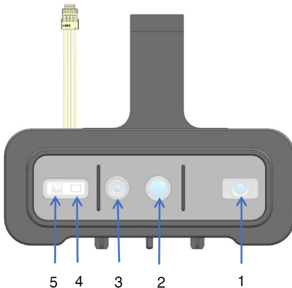
模块说明图 (编号对应系统组件表)
