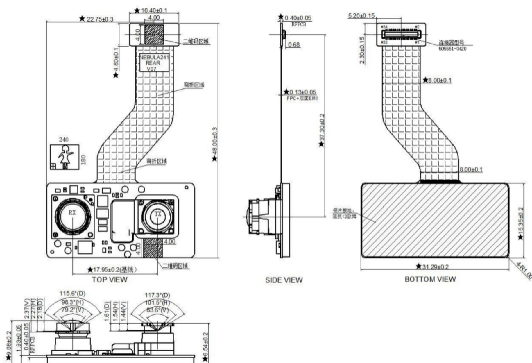
MIPI 模组尺寸结构图 (TOP / SIDE / BOTTOM VIEW, 含 FOV 标注与基线 17.95 mm)
