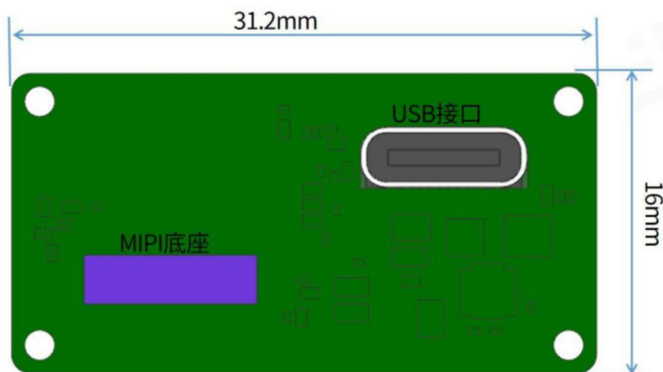
PCBA 尺寸结构图 (31.2 mm × 16 mm, 含 USB 接口与 MIPI 底座)
