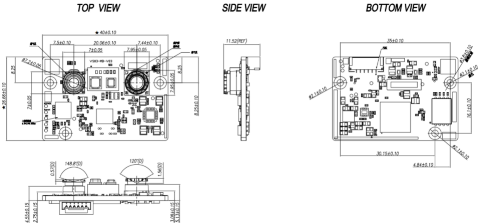
图：结构尺寸图
