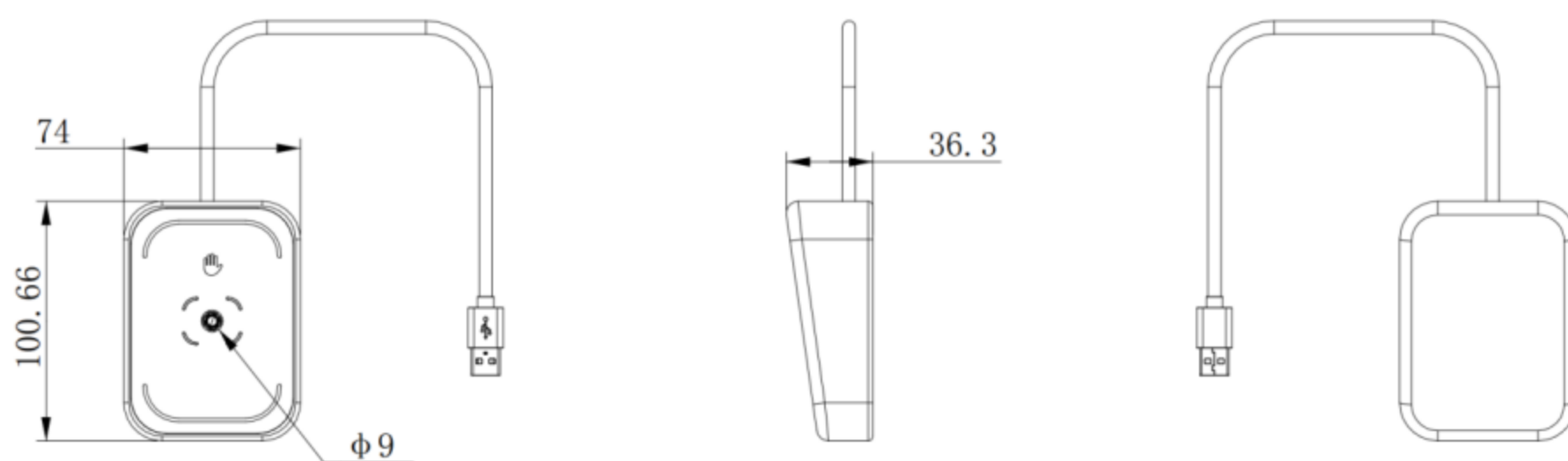
图：结构尺寸图
