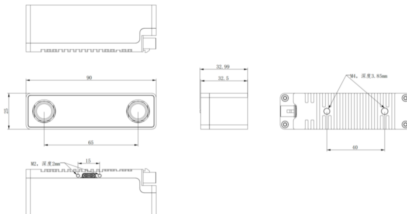
图：模组结构尺寸图 (90 × 25 × 32.99 mm)
