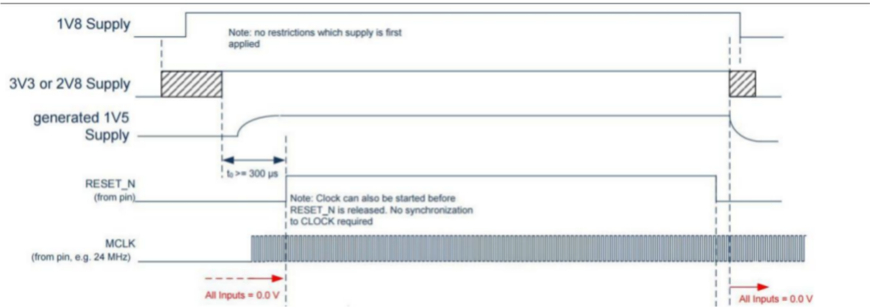
上电时序图（1V8 对应 DOVDD，3V3 对应 AVDD，1V5 为 Sensor 内部电压；5V 为激光器供电电压，在出流之前通电即可； t_0 \geq 300 \mu\text{s} ）
