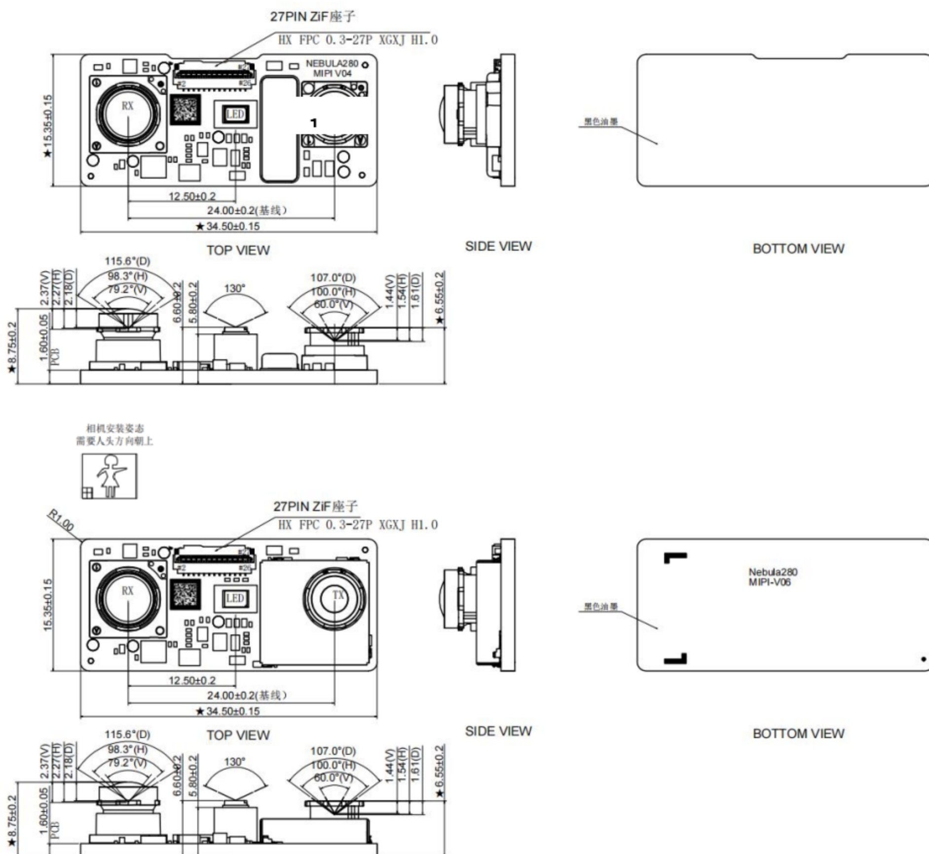
模组结构尺寸图 (TOP / SIDE / BOTTOM VIEW, 34.50 \pm 0.15 \times 15.35 \pm 0.15 mm, 基线 24.00 \pm 0.2 mm)
