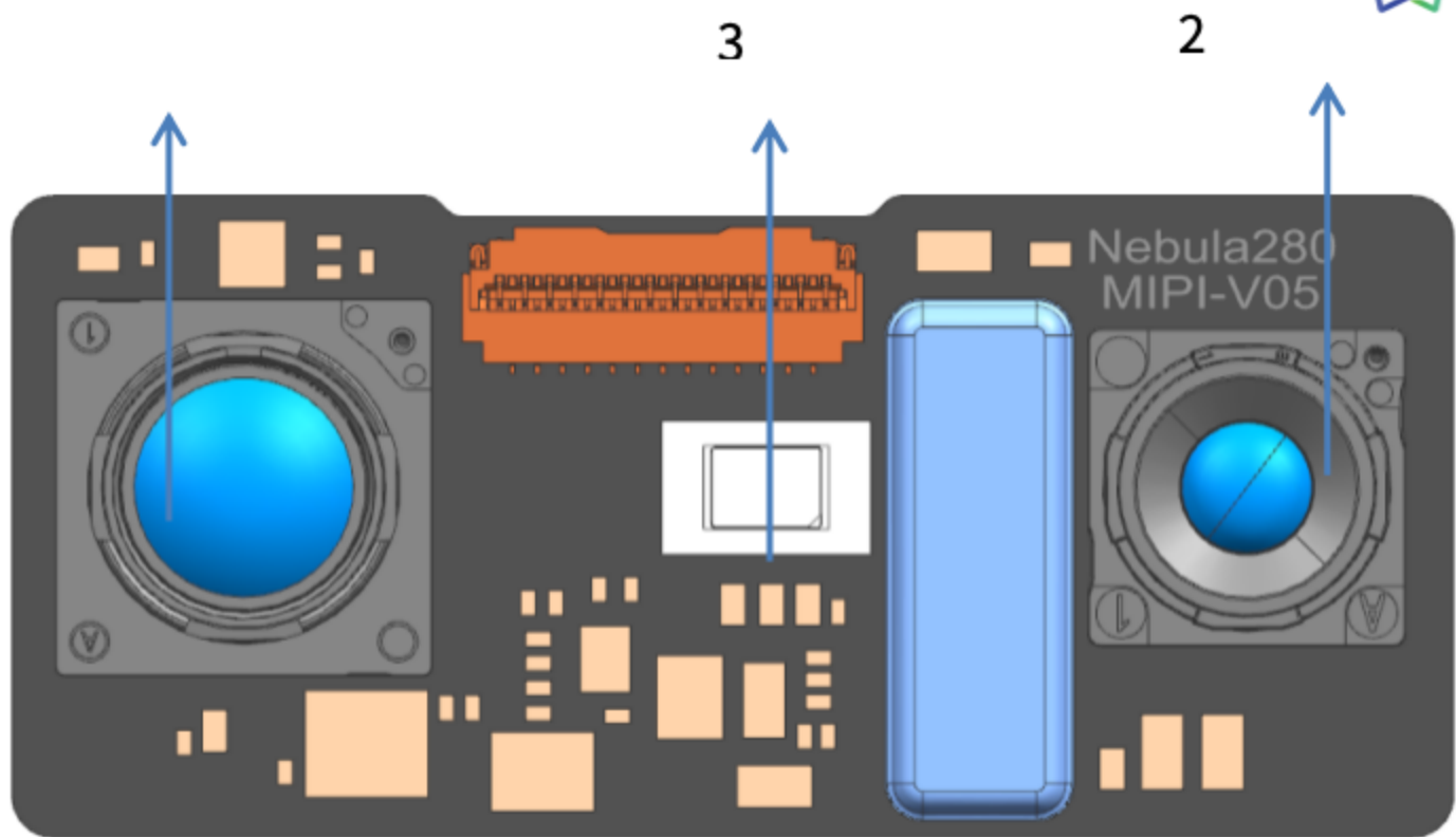
模块说明图（编号对应系统组件表）
