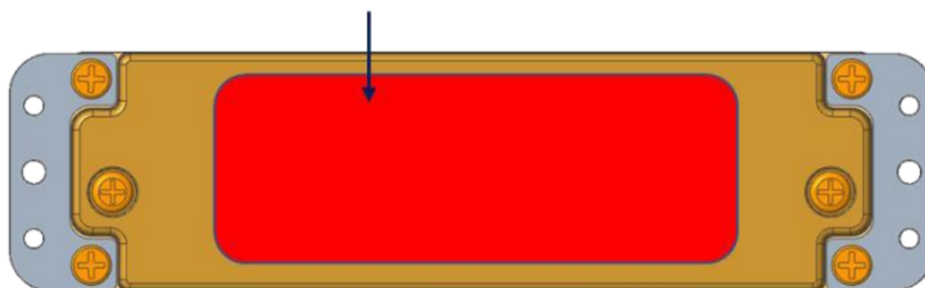
模组散热示意图（红色区域为导热硅胶贴附位置）
