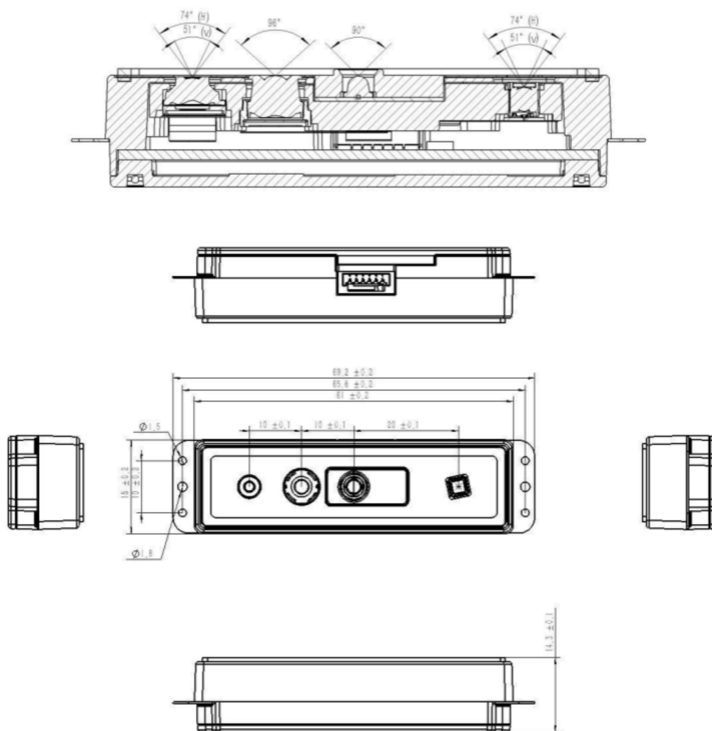
模组结构尺寸图 (L61 × W18 × H14.3 mm, 不含固定翼; 上图为各器件 FOV 剖面示意)
