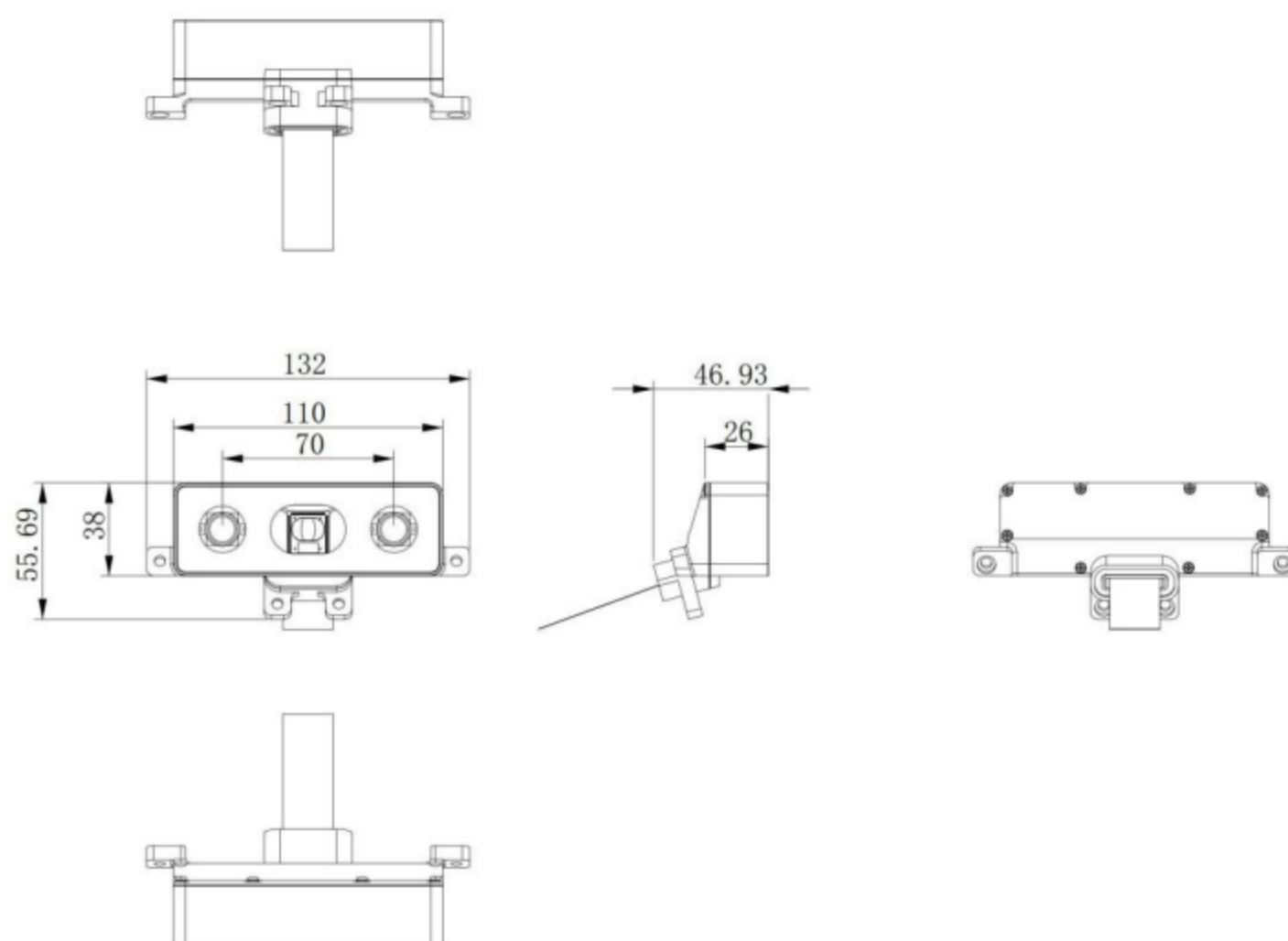
图：模组结构尺寸图 (132 × 55.69 × 46.93 mm)
